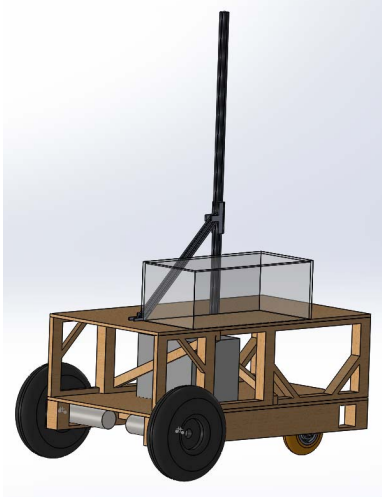
Fig. 1. CAD model of Eklavya 6.0.
